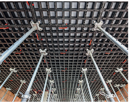
DUO 已針對厚度達 30 公分的樓板進行了優化。通用型 DFH 模板支撐頭可安裝在所有標準鋼管支撐上。
