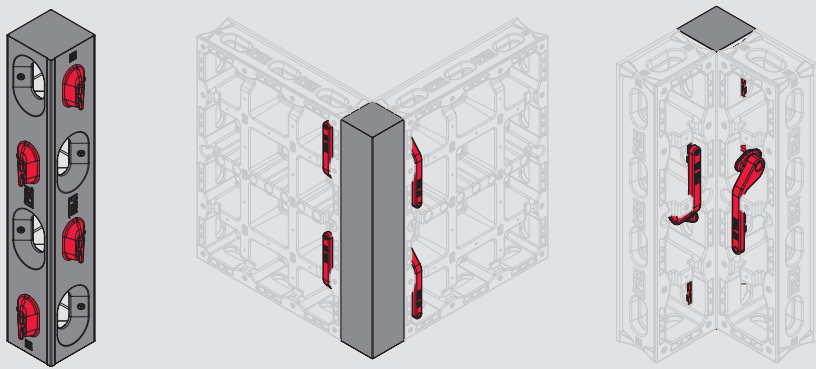
使用 DUO 鎖扣將角柱連接到 DUO 模板上。此示例展示了內角和外角兩種應用方式。
