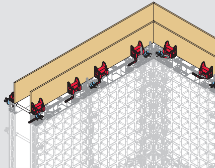
對於最高 30 公分的定制化高度增高, 可以選擇安裝 DUO 高度延伸器。這些高度延伸器可以放置在任意模板上。
