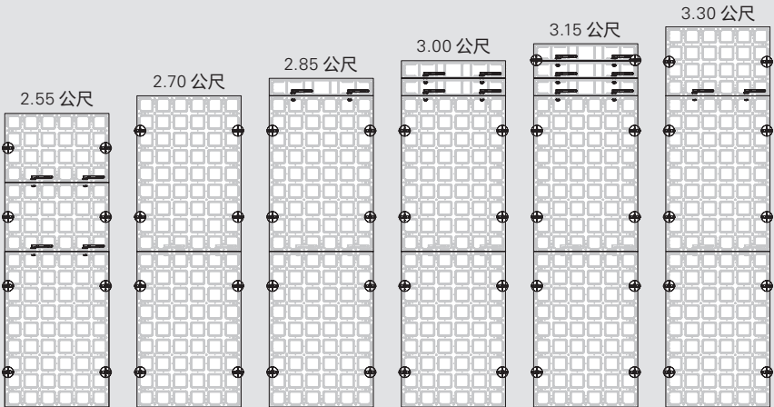
通過組合 135 公分和 0.60 公尺高的模板, 可以實現 2.55 公尺、2.70 公尺和 3.30 公尺的牆高。如果在擴展時額外使用 15 公分的增高模板, 則可以將高度調節靈活性最大化。
