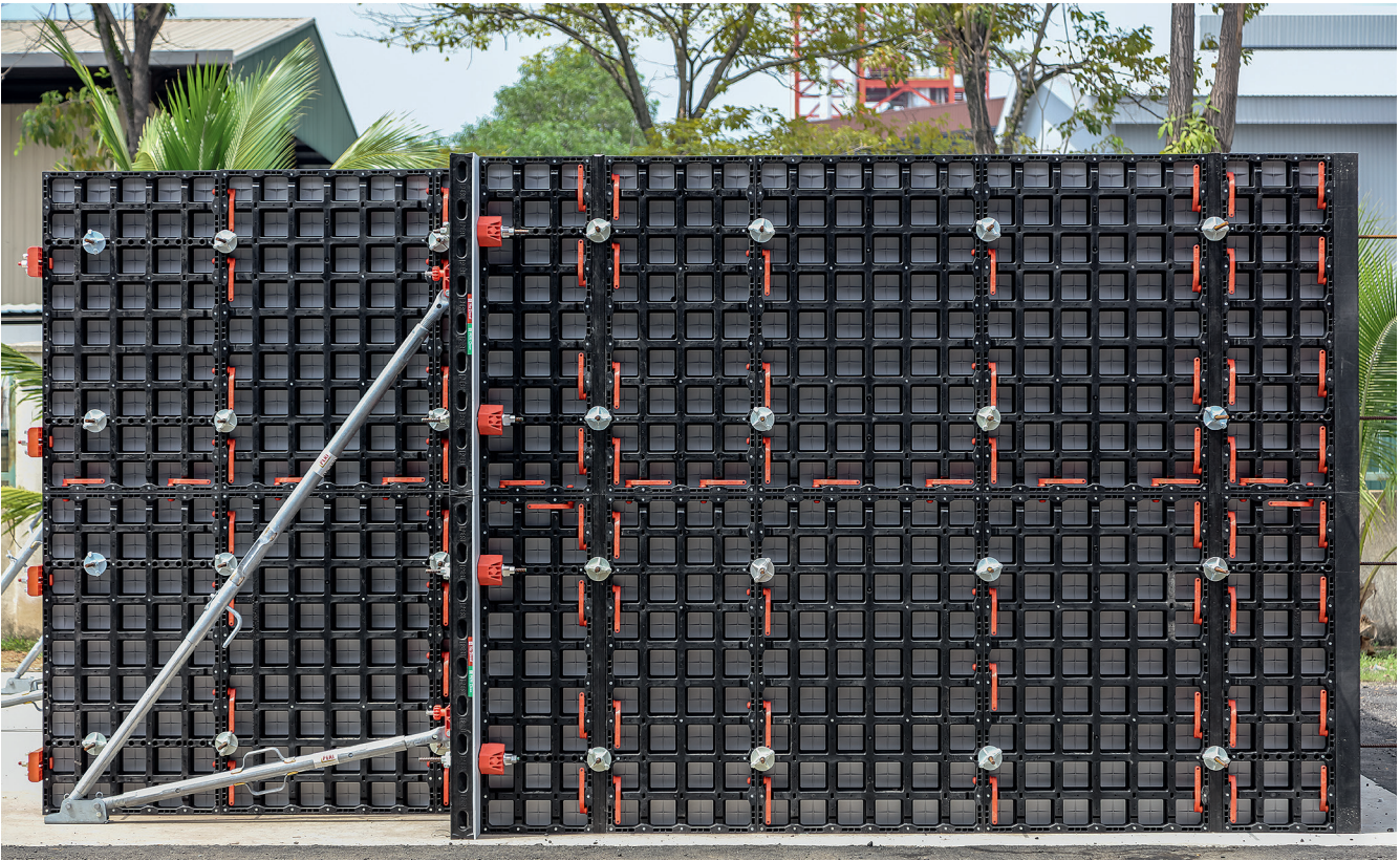
DUO 已針對 2.7 公尺的樓層高度進行了優化 - 在每種情況下使用 2 個標準面板實現延伸。結合橫向延伸的可能性以及 60 公分高的可用面板, 將帶來無數的可能性。
