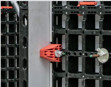
.....然後將螺桿穿過多功能模板上的連接孔固定。
