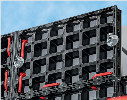
可以任意組合高度為 1.35 公尺和 0.60 公尺的標準面板, 來為牆模的高度調節提供廣泛的可能性。
