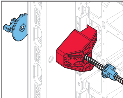
通過轉角連接器和轉角連結螺桿，以 5 公分為增量將兩個多功能模板呈直角連接在一起。
